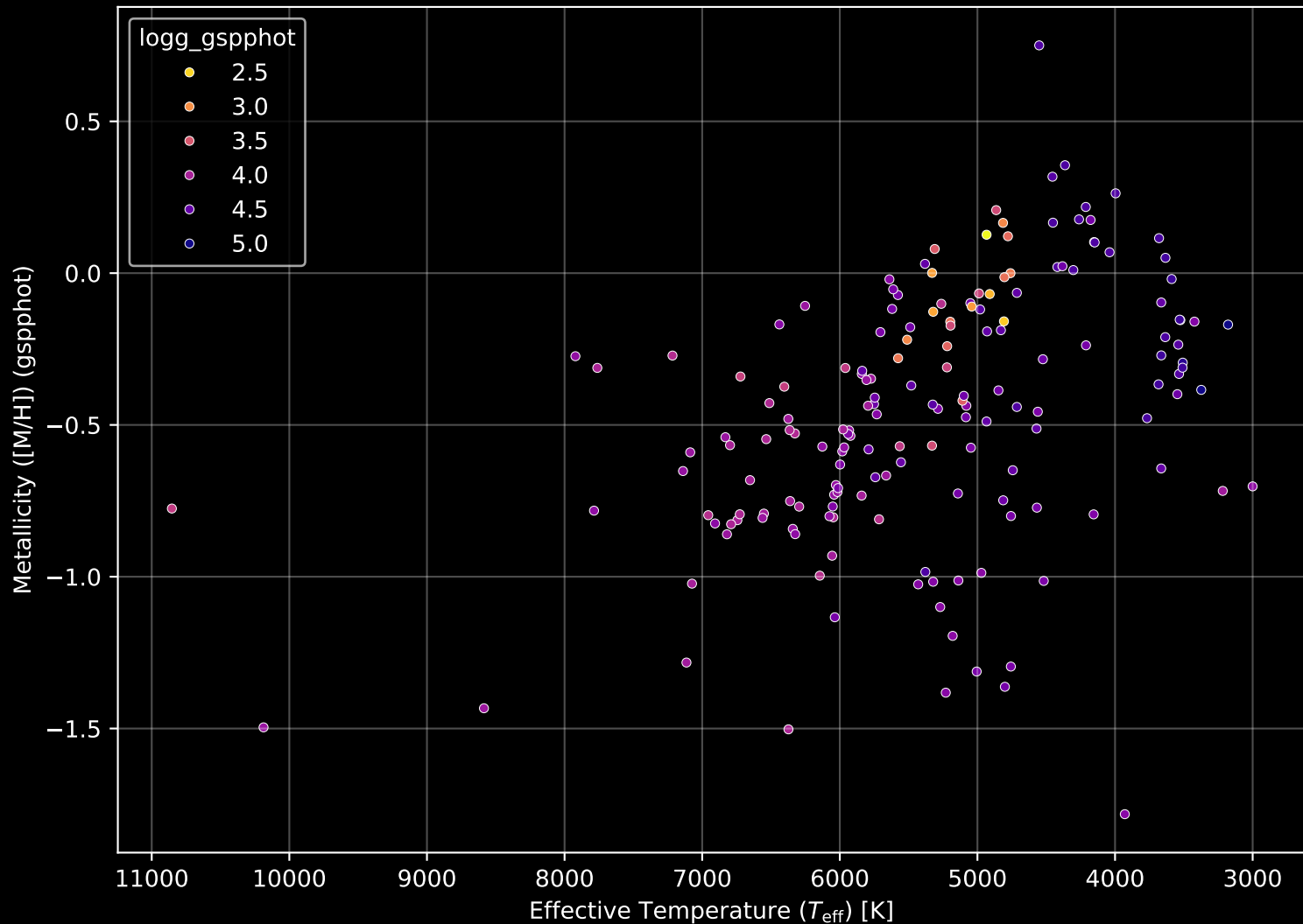
APOGEE DR17 Field: [K2_C13_178-20_btx] Stellar Population Parameters (n= 172)
